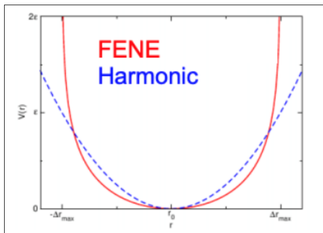
Figura 7: Curve di potenziale del modello ad armoniche e FENE
